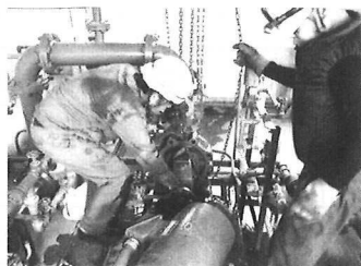
ポンプ分解整備(浜忠地区)
